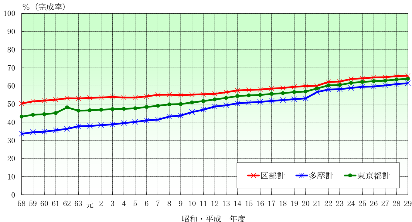
図表 1－5－3 都市計画道路の整備状況
