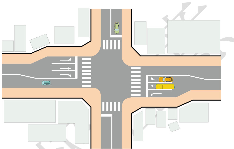
図-24 交差点拡幅部のイメージ
