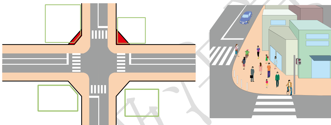
図-26 隅切りのイメージ
