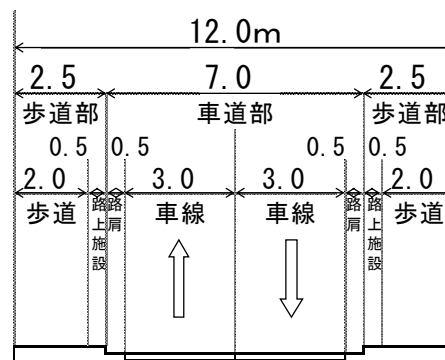
図 3-52 地域的な道路の評価幅員の例
