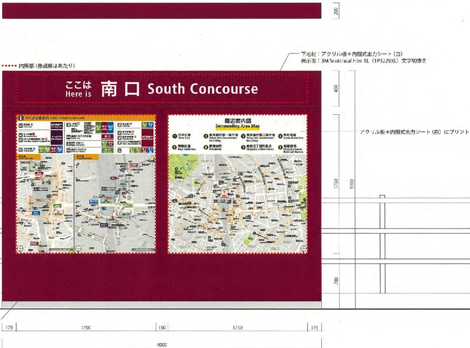
KK-図01 器具外形寸法H3000×W4000 (タイトル和文文字高200)
