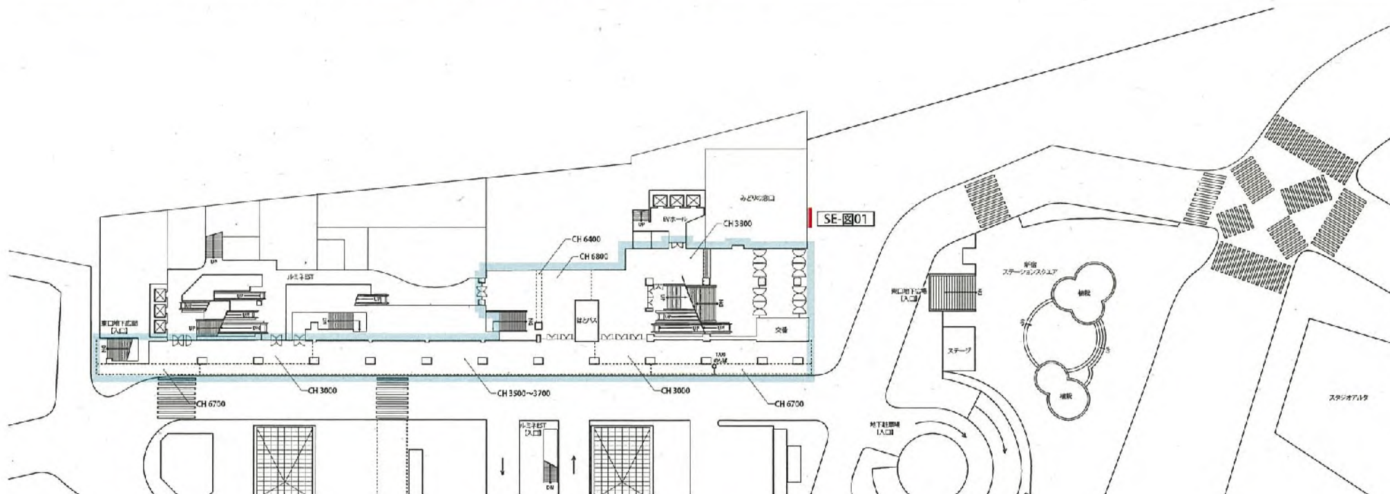
SE-図01 ターミナルマップ+エアリアマップ
