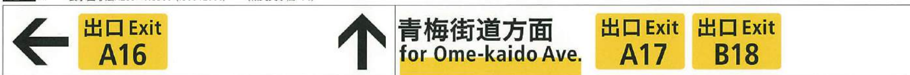
M①-06 -a 表示面寸法H280×W3500 (1500+2000) (和文文字高: 90)
