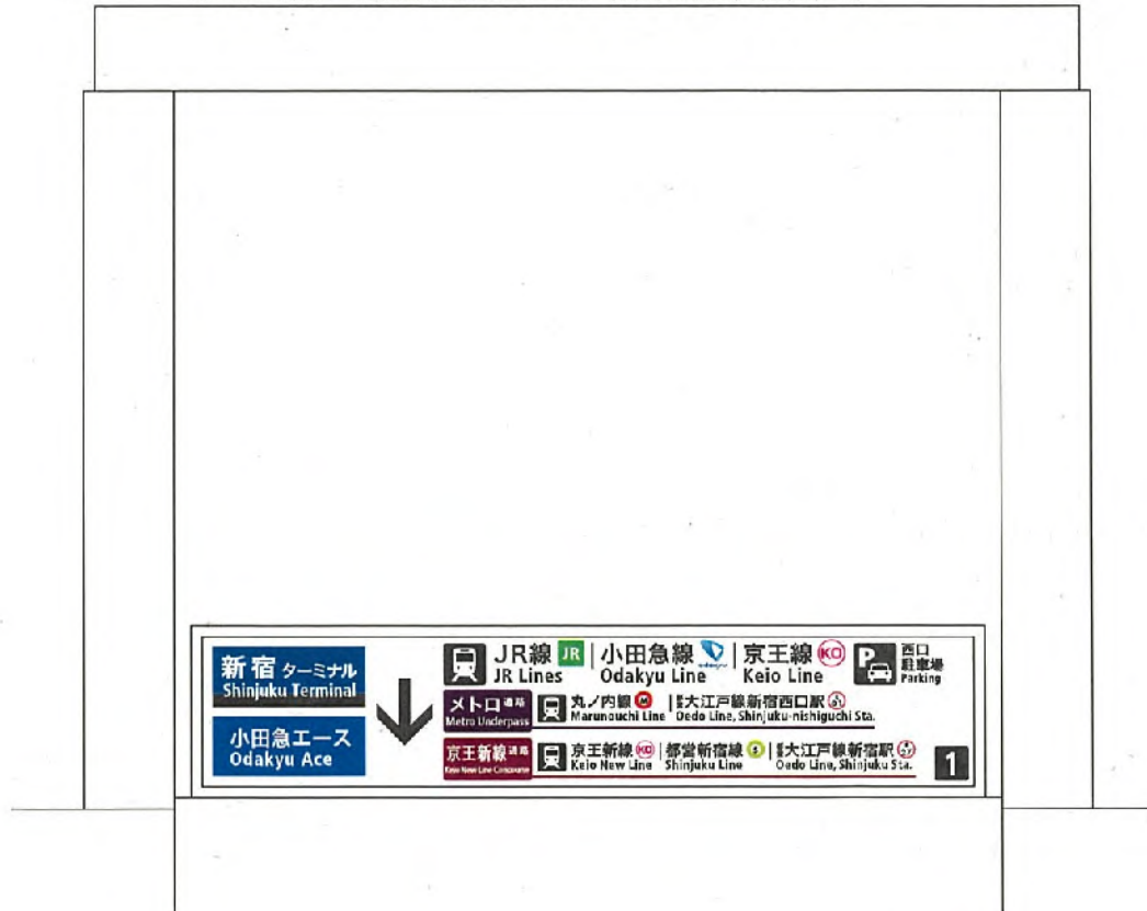
西-4001<片面> 表示面寸法H530×W2730 (和文文字高81,75,72,50,45.5)
