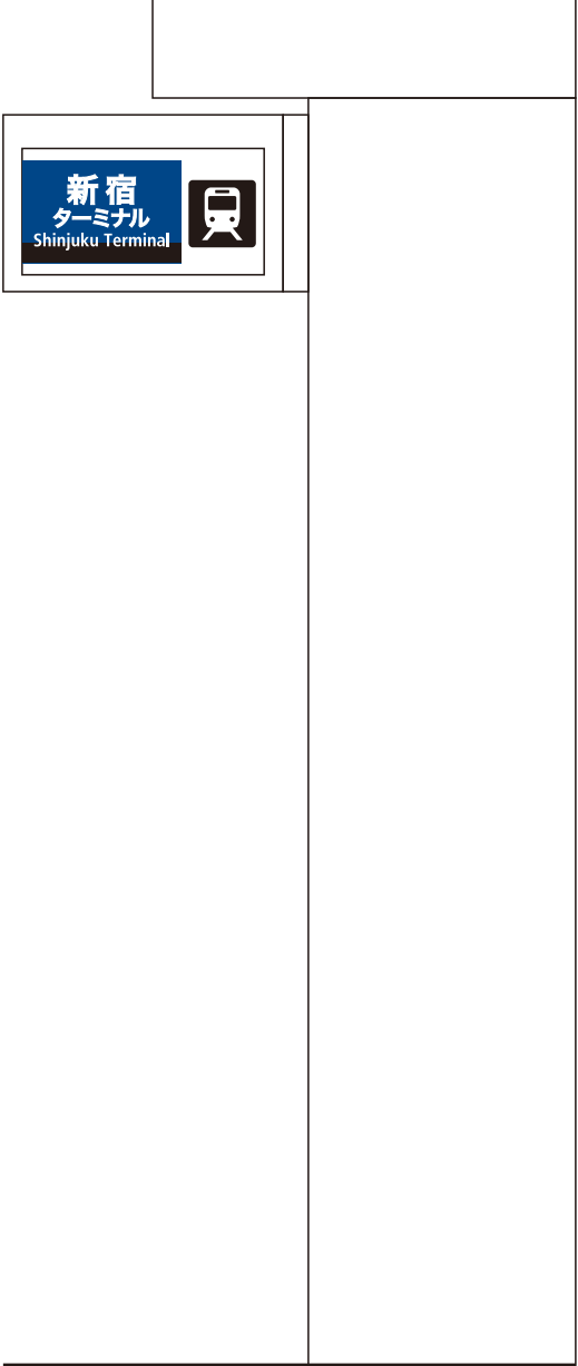
西-2002＜両面＞ 表示面寸法H300×W575（新宿文字高70）
