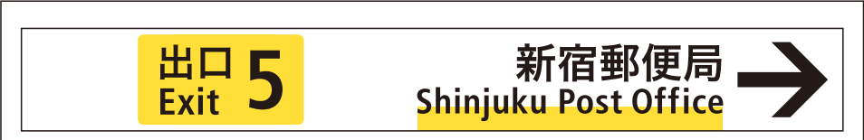
西-2009<両面>ウラ 表示面寸法H300×W2430 (和文文字高110)
