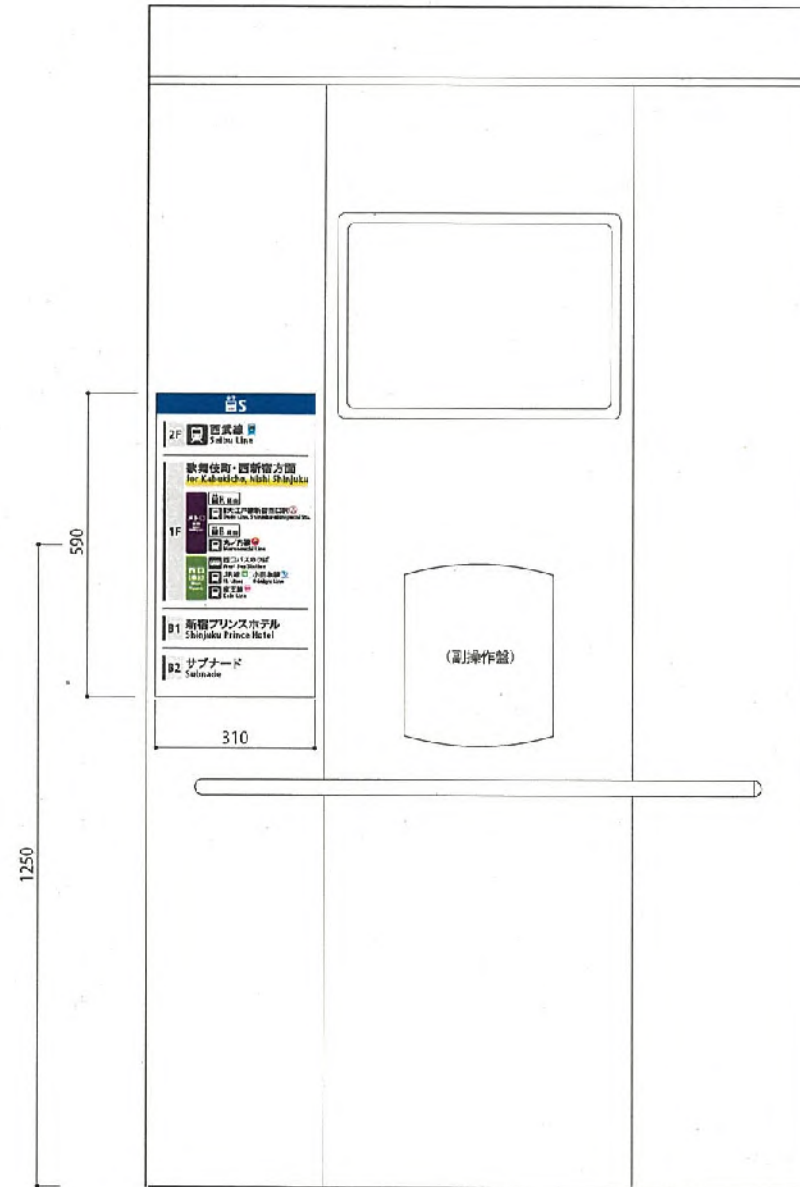
EV-S02 S=1/10
