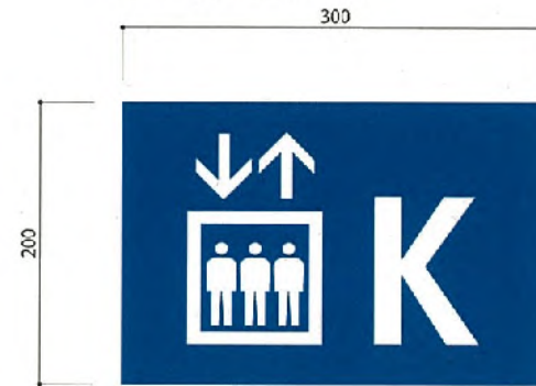
EV-K01 拡大図 (S=1/4)
