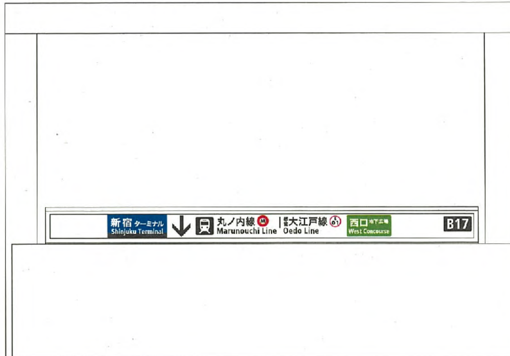
西-3015<片面> 表示面寸法H190×W3330 (和文文字高70)
