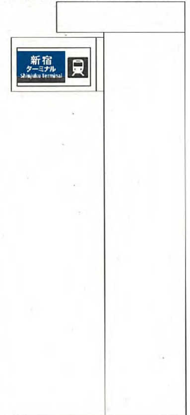
西-2002<両面> 表示面寸法H300×W575 (新宿文字高70)
