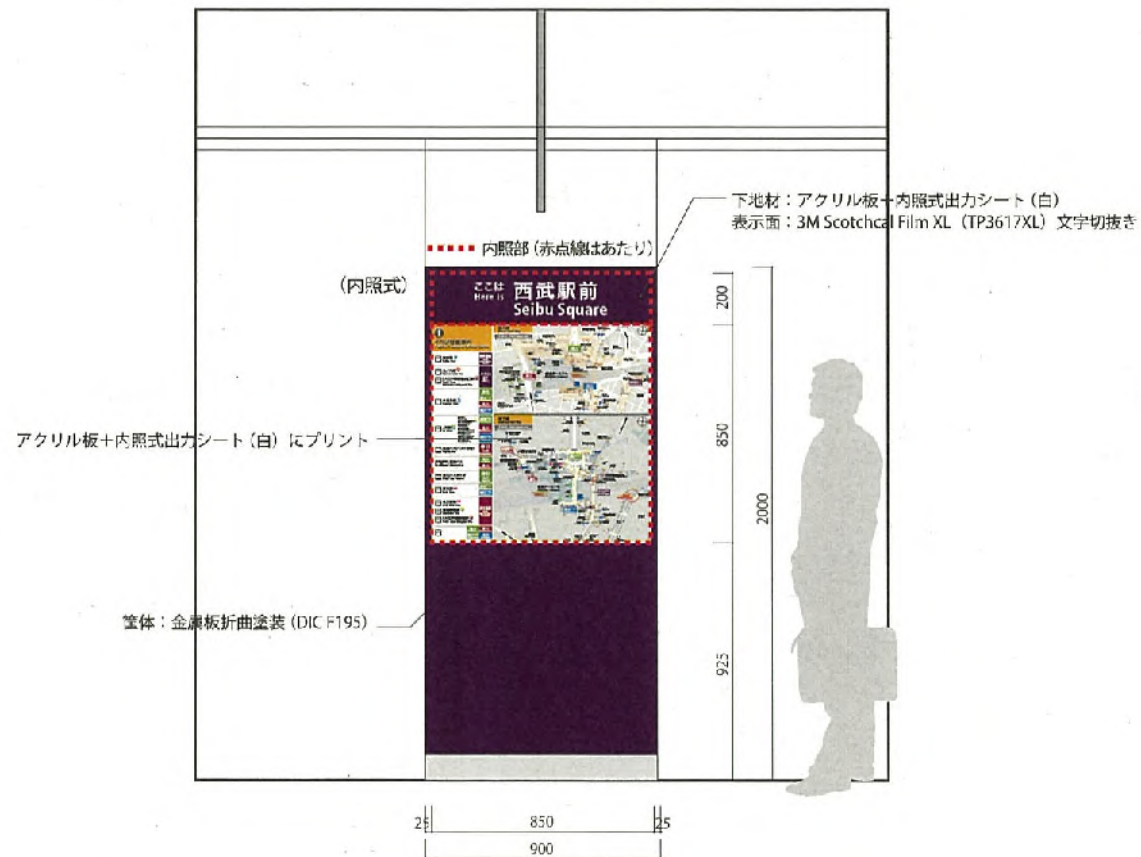
SN-図01 器具外形寸法H2000×W900 (タイトル和文文字高70)
