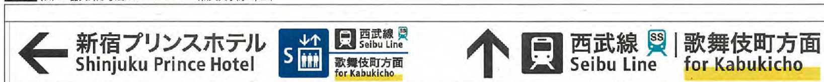
SN-02 (新)-b 器具外形寸法H470×W4800 (和文文字高60,120)
