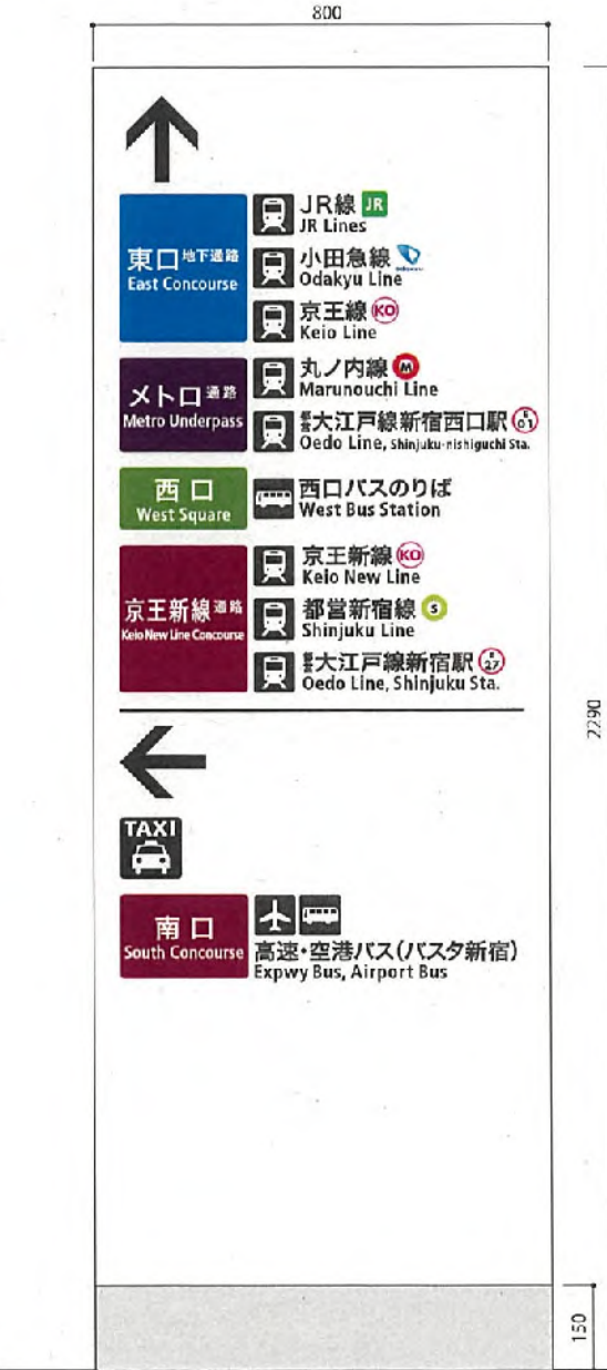
J①'-13 器具外形寸法H2290×W800 (和文文字高36)
