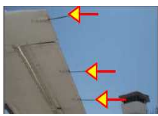
スタティックディスチャージャー(放電索)
