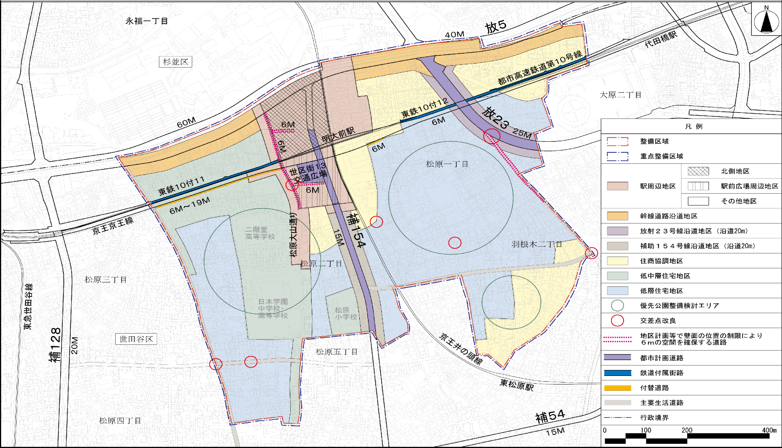
A16-054 明大前駅周辺地区住宅市街地総合整備事業(密集型)
