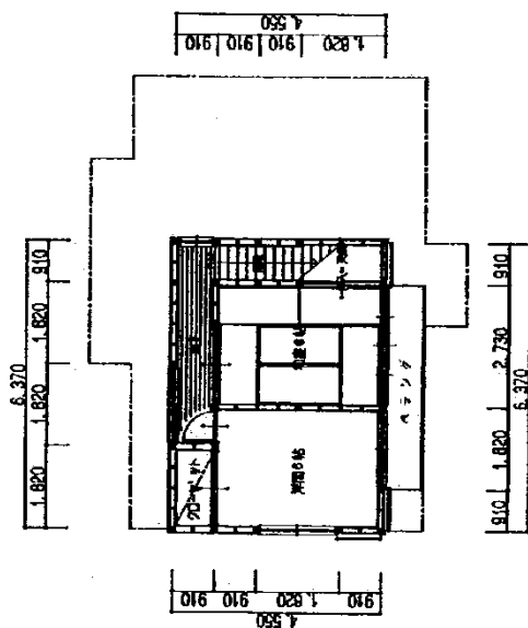
2階平面詳細図 S=1/100
