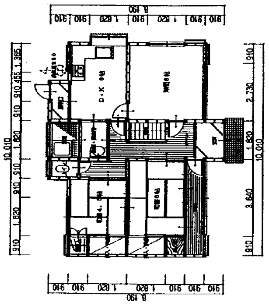
1階平面詳細図 S=1/100
