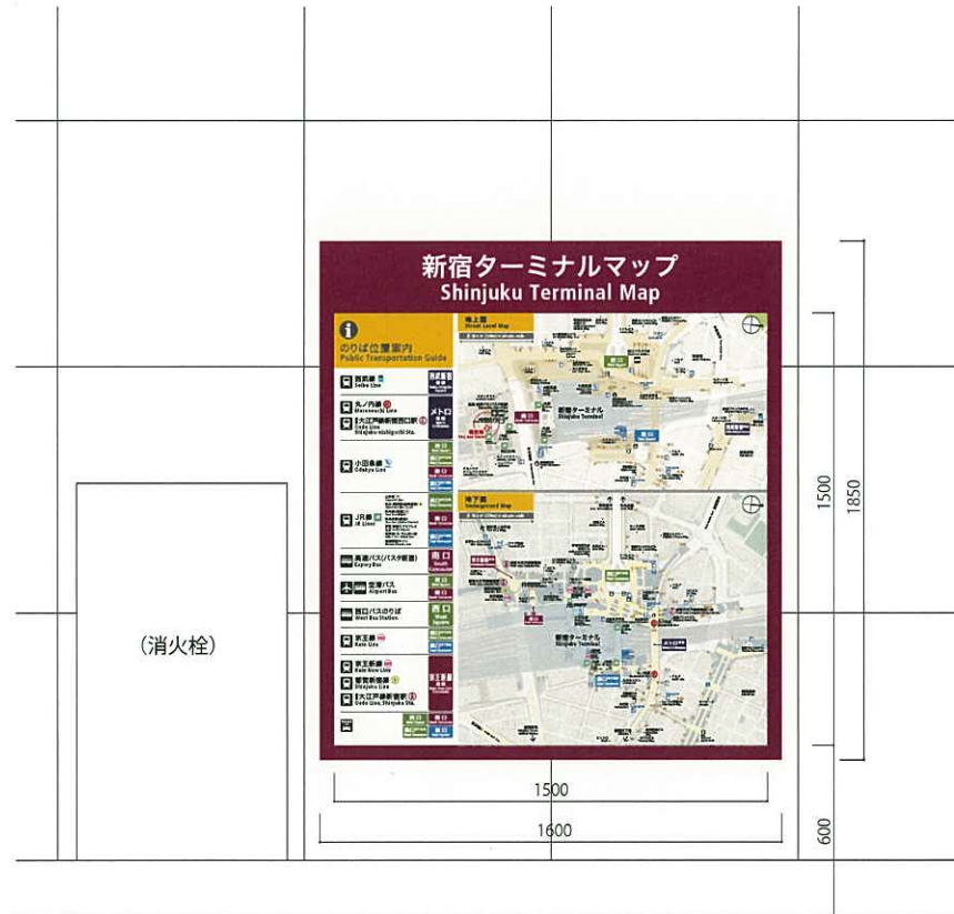
B-図03 器具外形寸法H1800×W1600
