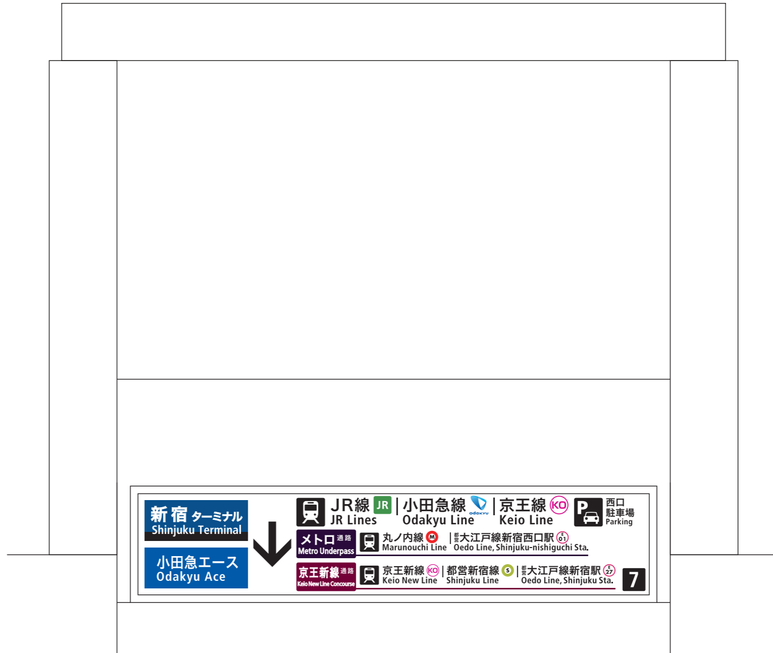
西-7001<片面> 表示面寸法H530×W2680 (和文文字高81,75,72,50,45.5)
