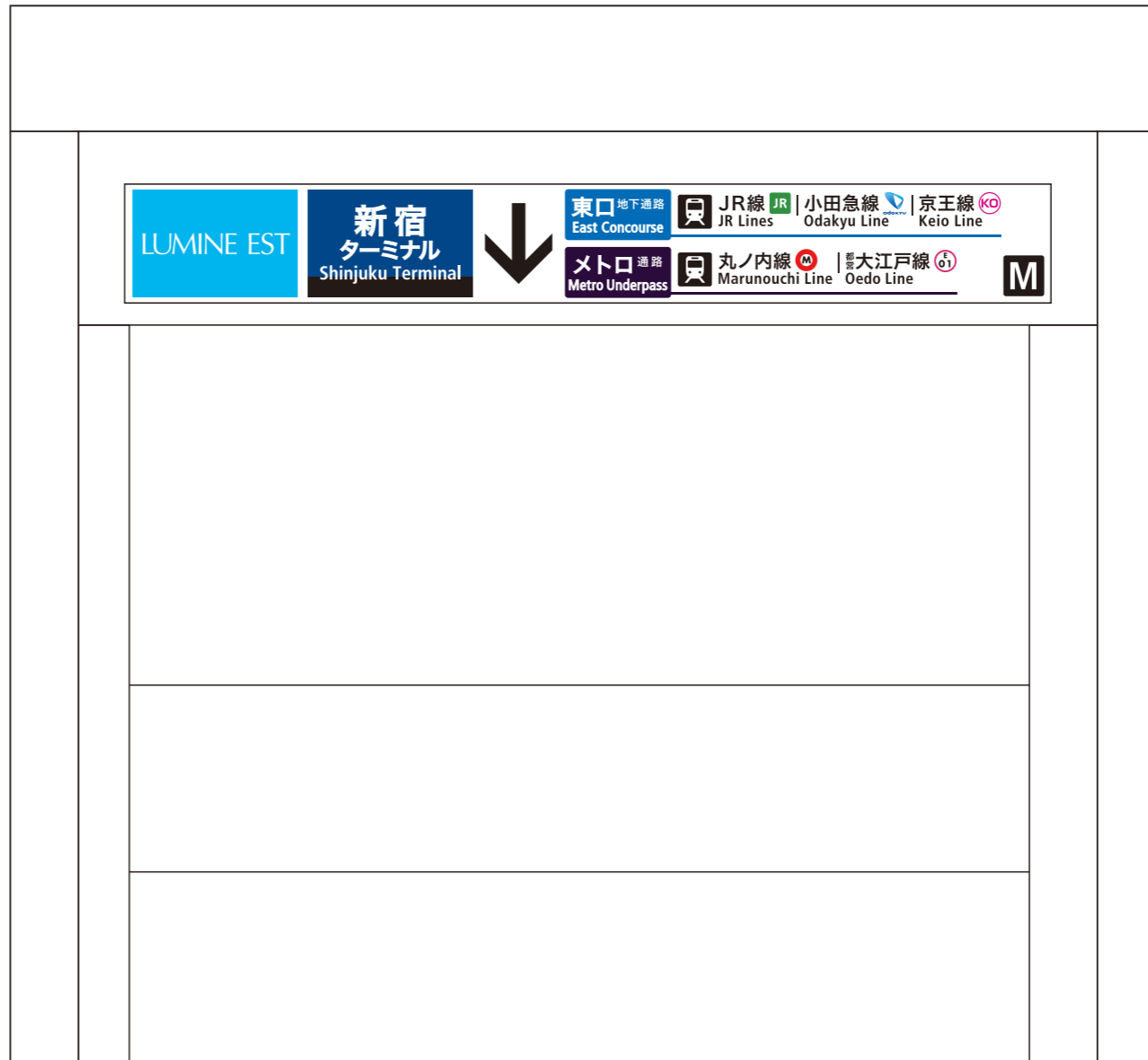
東-6011<片面> 表示面寸法H350×W2730 (和文文字高90,50)
