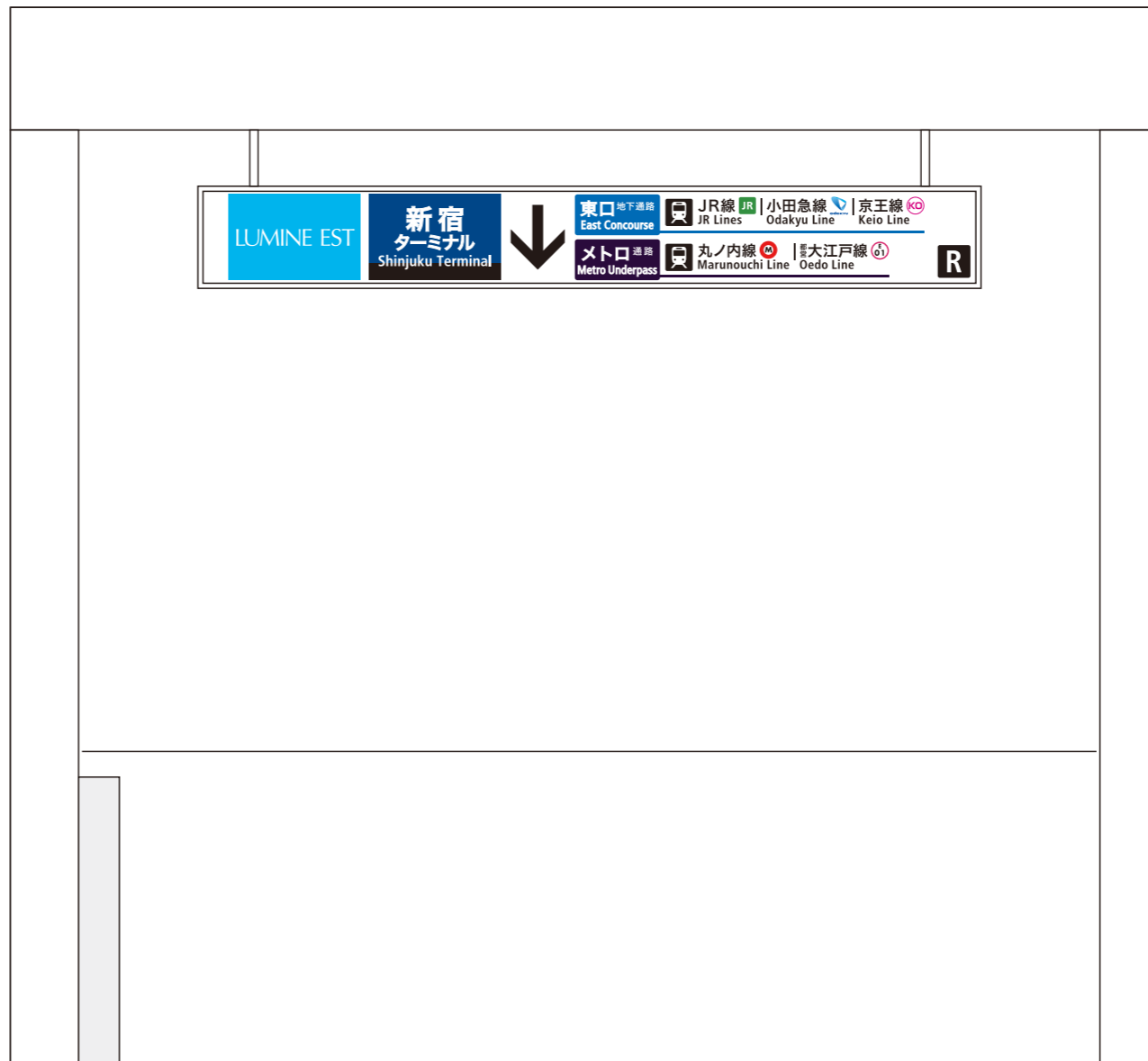
東-6006<両面> 器具寸法H300×W2300 表示面寸法H270×W2270 (和文文字高72,40)
