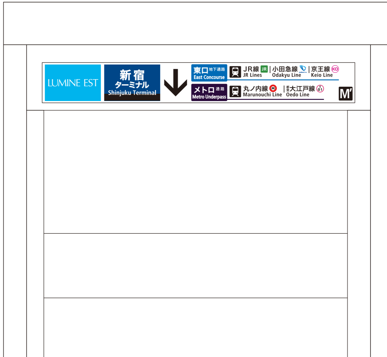
東-6010<片面> 表示面寸法H350×W2720 (和文文字高90,50)
