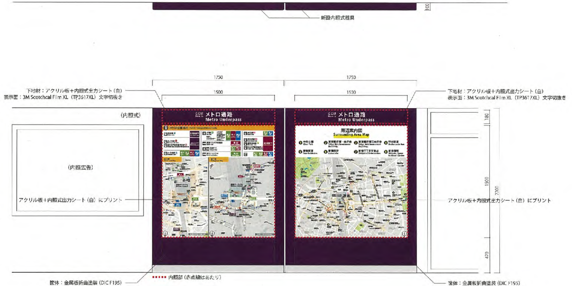
M②-図03 器具外形寸法H2200×W1750 (タイトル和文文字高65)
