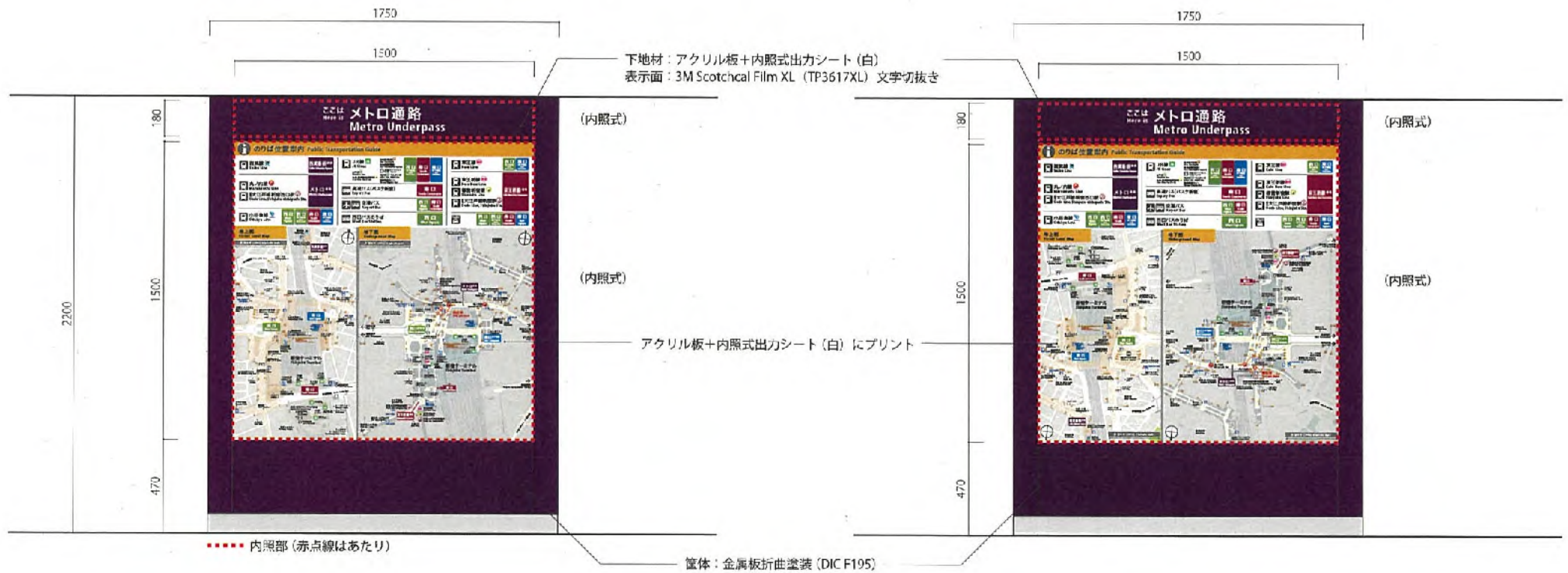
M②-図02 器具外形寸法H2200×W1750 (タイトル和文文字高65)
