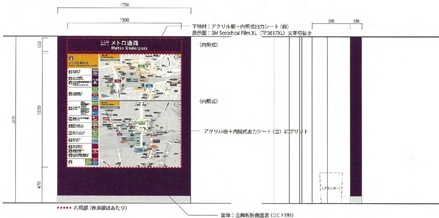
M②-図01 器具外形寸法H2200×W1750 (タイトル和文文字高65)
