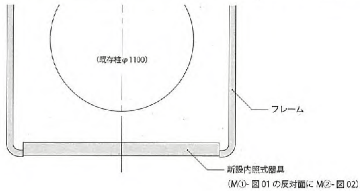
M①-図01 器具外形寸法H2200×W1750 (タイトル和文文字高65)
