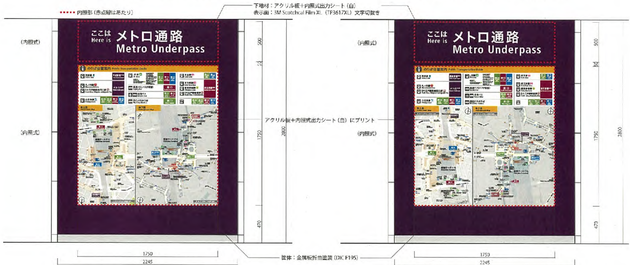
M①-図04 器具外形寸法H2800×W2245 (タイトル和文文字高150)
