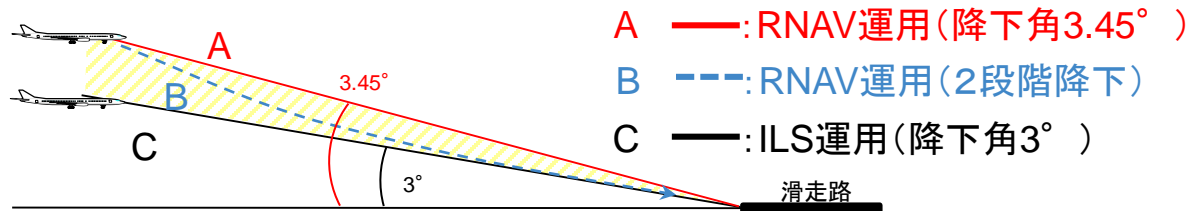
<RNAV運用(3.45度降下)と2段階降下のイメージ図>
