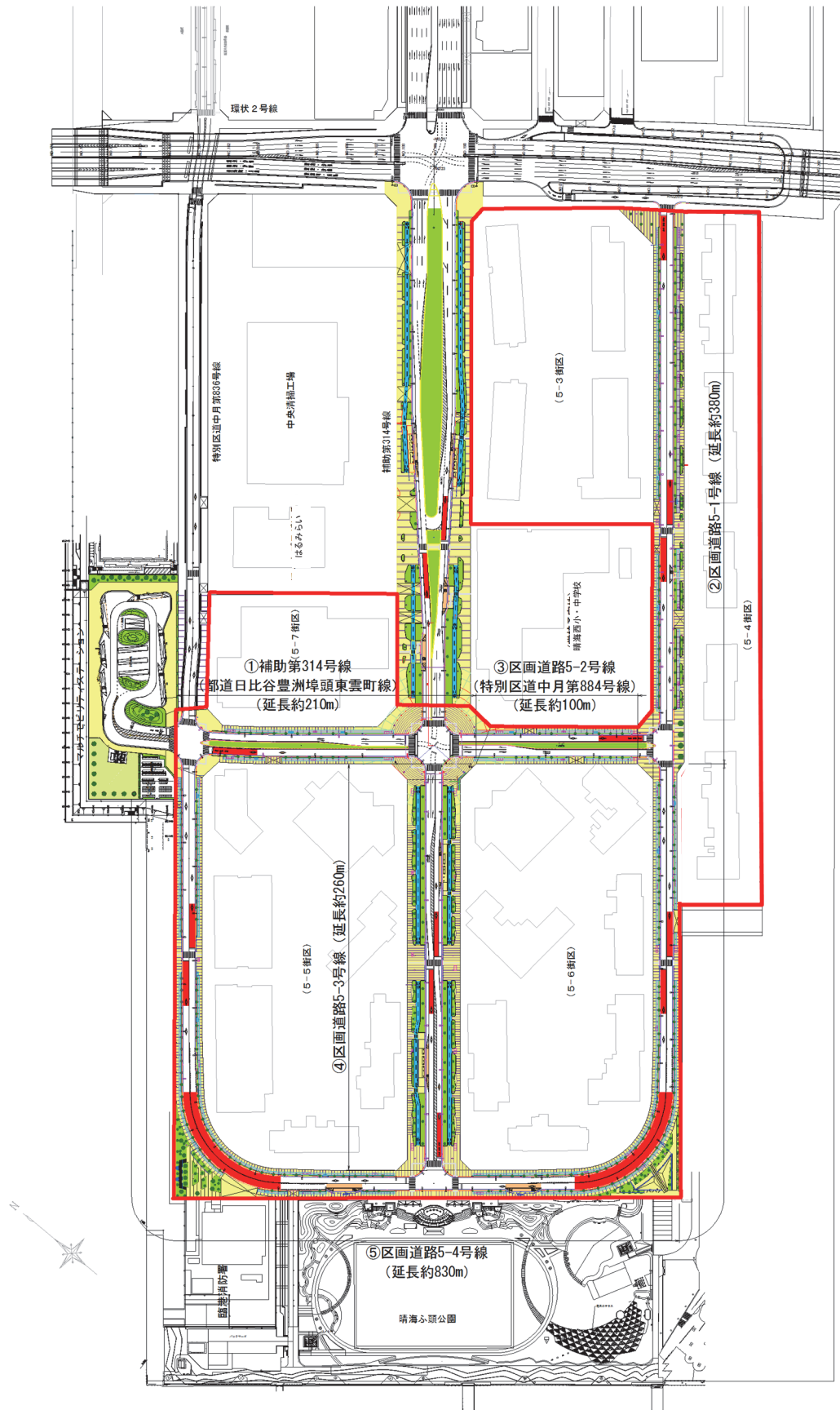
図3 道路平面図
