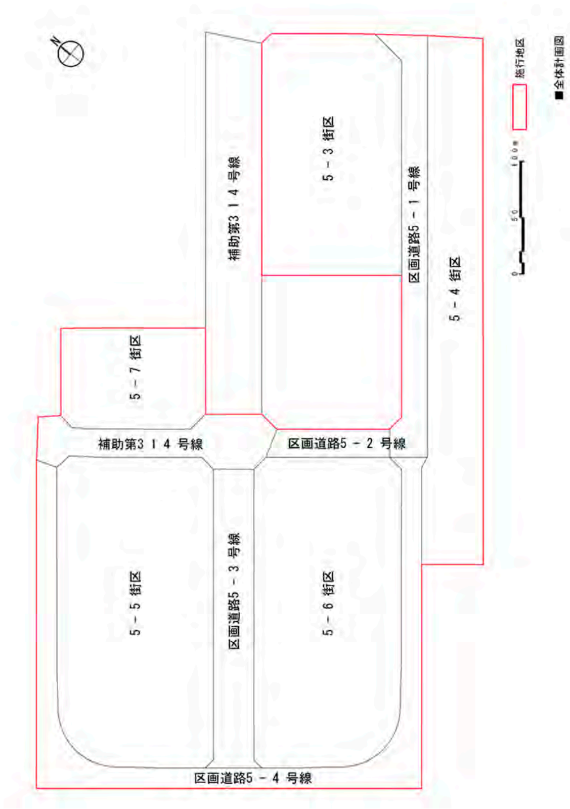
図1 全体計画図
