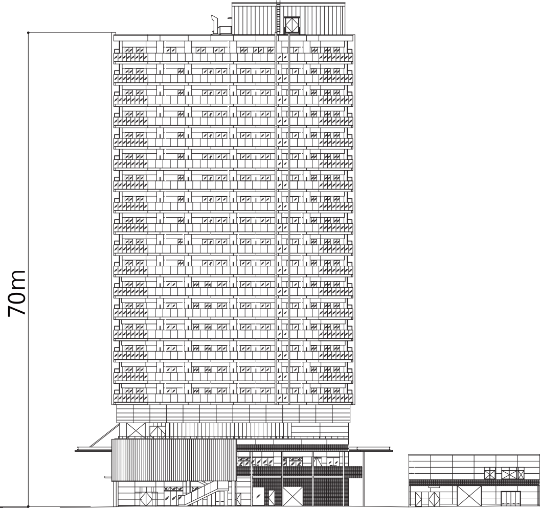
2 東側立面図 1/600
