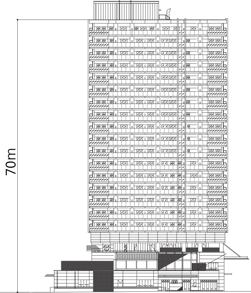
4 西側立面図 1/600 0m 5m 10m 20m 30m
