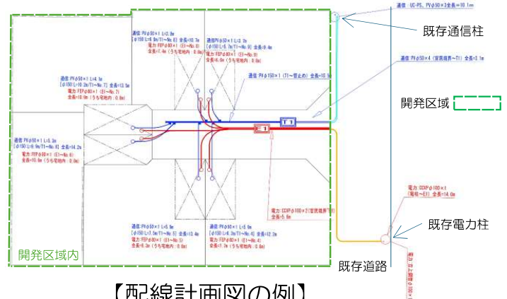
【配線計画図の例】
