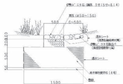
- 断面図 -
