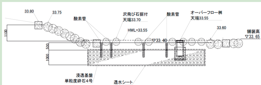
- 断面図 -
