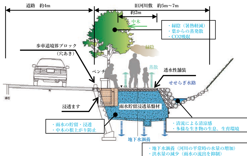
- 断面図 (Cゾーン) -
