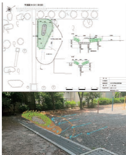
- 雨庭Aの検討 -
