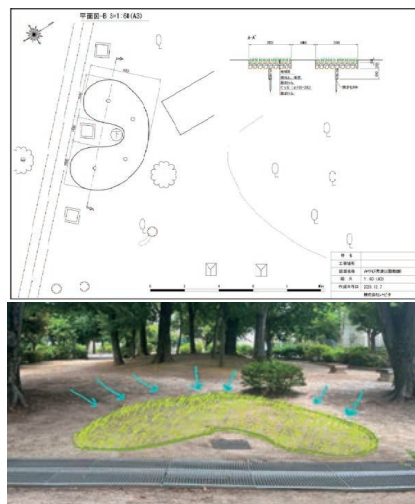
- 雨庭Bの検討 -
