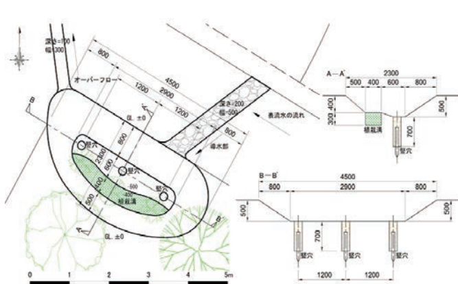
- 施工図 -
