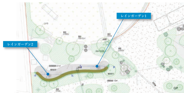
- 計画平面図 -
