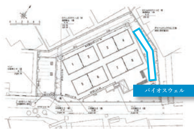
- 計画平面図 -
