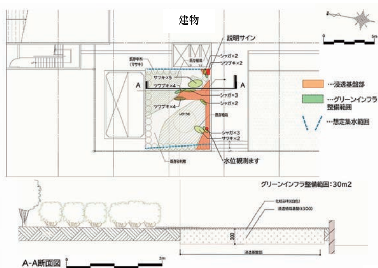
- 竣工図 -
