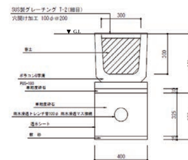
- 雨水浸透設備断面図 -
