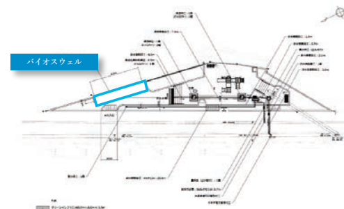
- 計画平面図 -
