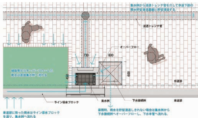
- グリーンインフラシステム概要図 -
