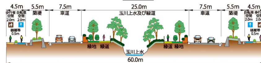
横断図
