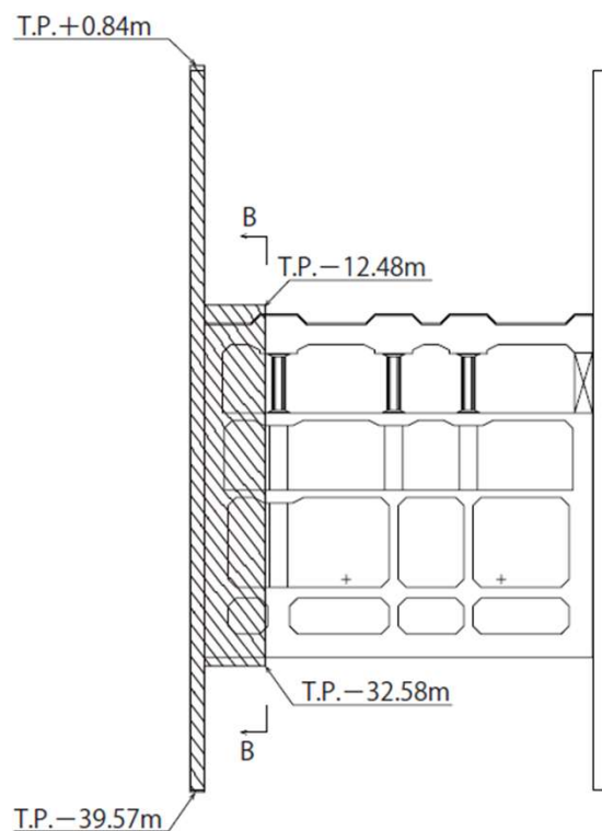
横断面図 A-A 断面図
