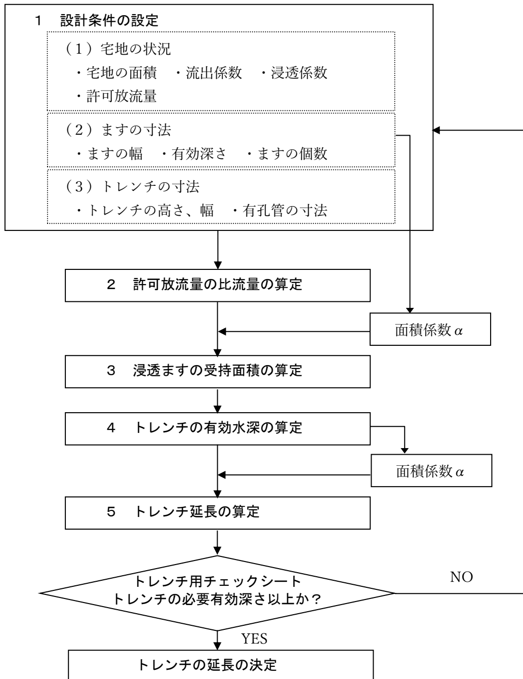
トレンチの計算手順フロー
