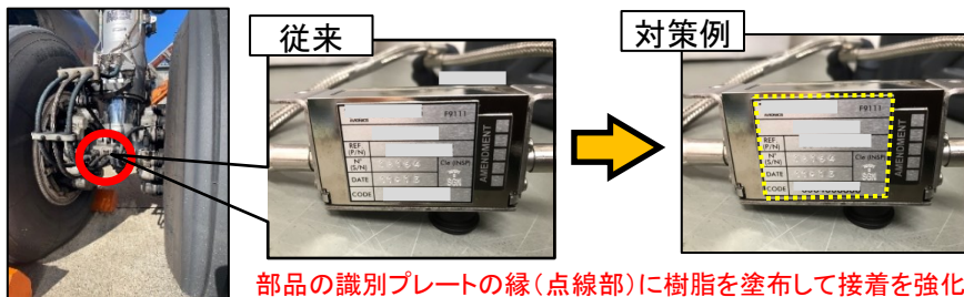
部品の識別プレートの縁(点線部)に樹脂を塗布して接着を強化
