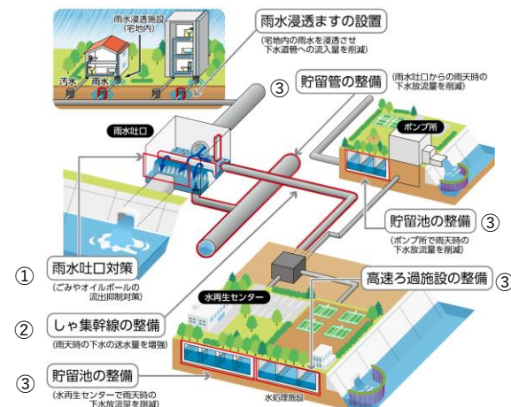
図 日本橋川流域における下水道施設の現況
