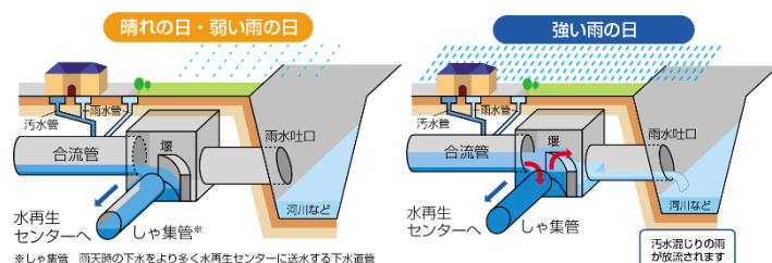
図 合流式下水道の特徴
