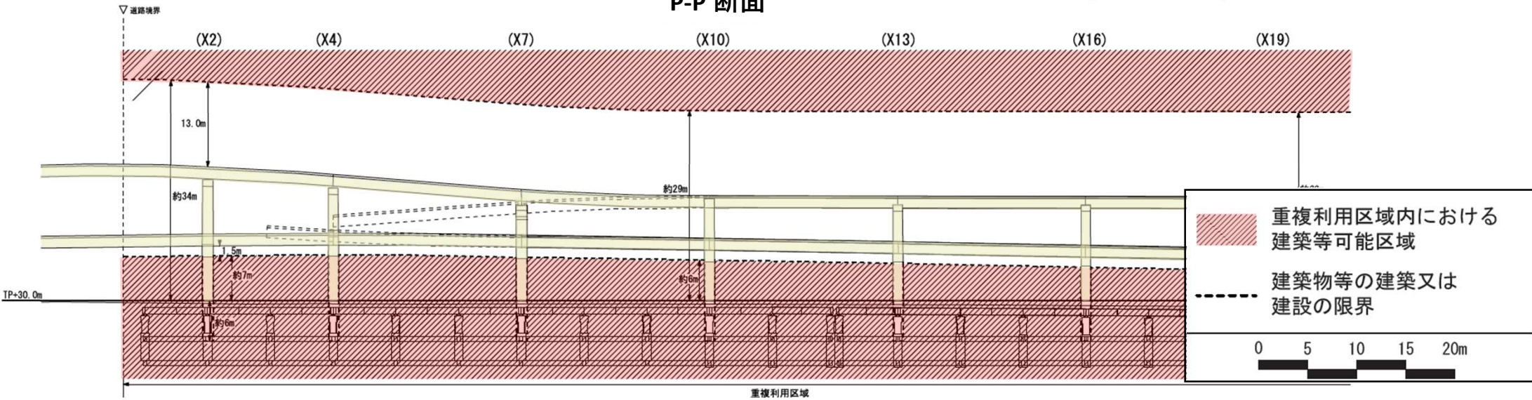
P-P'断面
