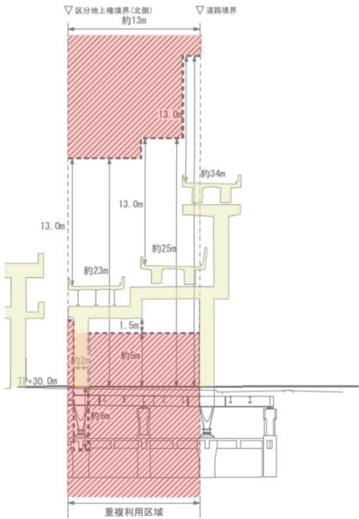
A-A'断面
