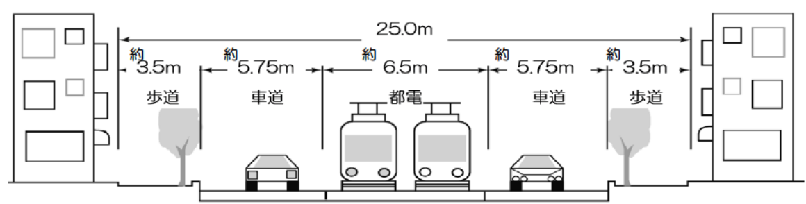
道路の構造（標準断面）
