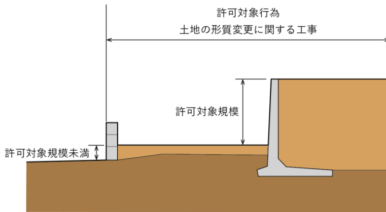
図 1-24 不陸整正など許可対象規模未満の造成を含む宅地造成のイメージ
