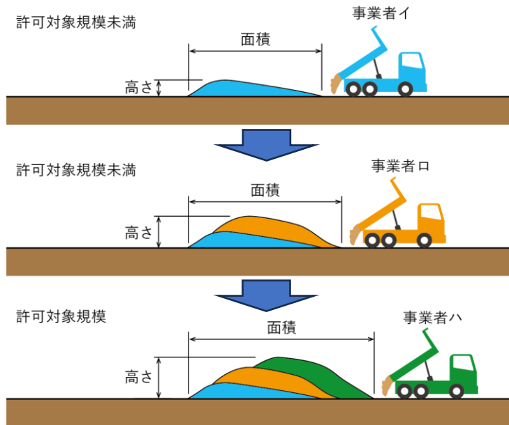
図 1-29 繰返し行われる土石の堆積の一体性
