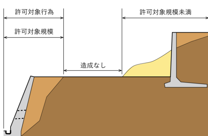
図 1-19 造成がない土地に隣接して行われる許可対象行為の考え方
