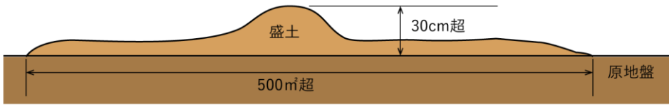
図 1-21 盛土又は切土する土地の面積が 500m 2 超で、盛土又は切土をする前後の地盤面の標高の差が 30cm 超となる場合イメージ
