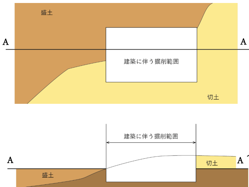
図 1-23 盛土等をする土地の面積における建築に伴う掘削範囲の取扱
