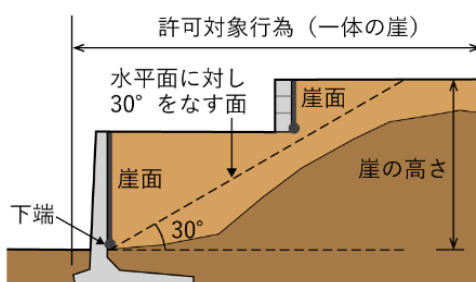
図 12 崖の高さ (一体の崖)
