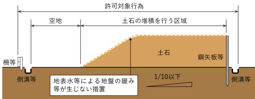
図 1-27 許可対象行為となる土石の堆積
