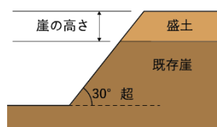
図 10 崖の高さ (盛土)
