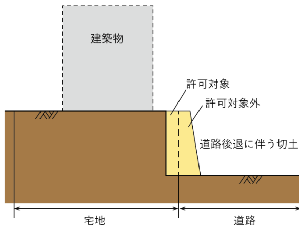
図 1-25 道路後退に伴う造成の許可対象行為となる範囲
