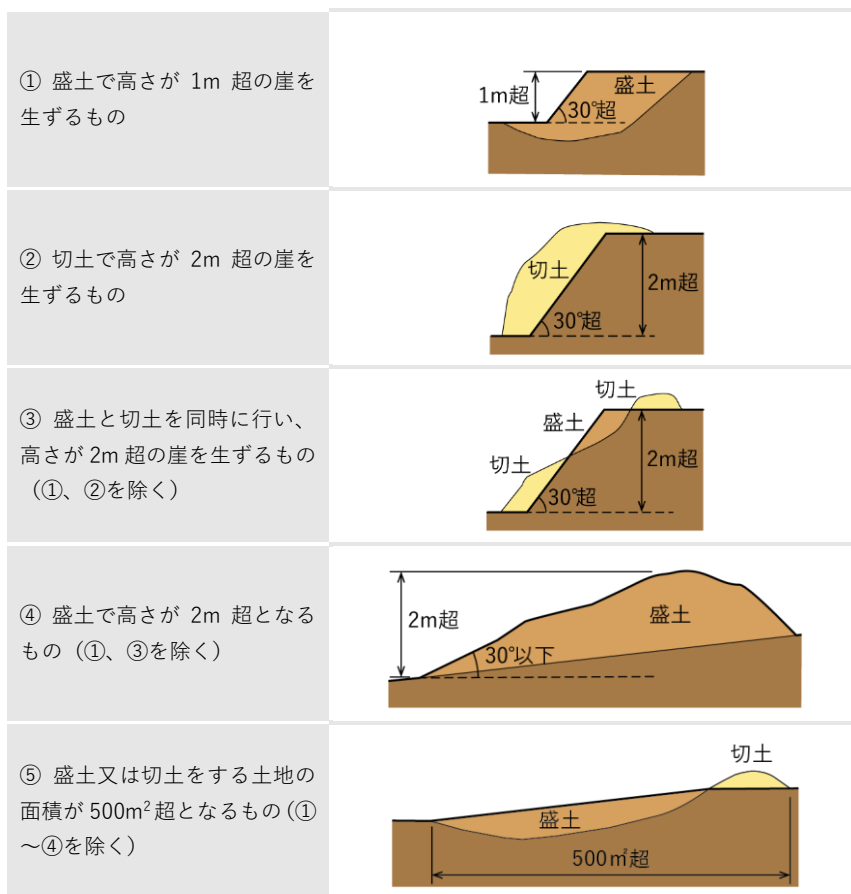
図 1-3 土地の形質の変更(盛土・切土)の定義
