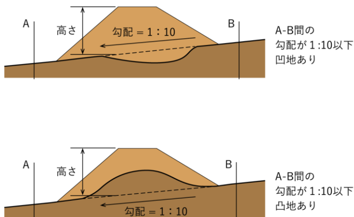
図 1-28 堆積地盤の一部に凹凸がある場合の堆積高さの考え方
