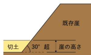
図 11 崖の高さ (切土)
