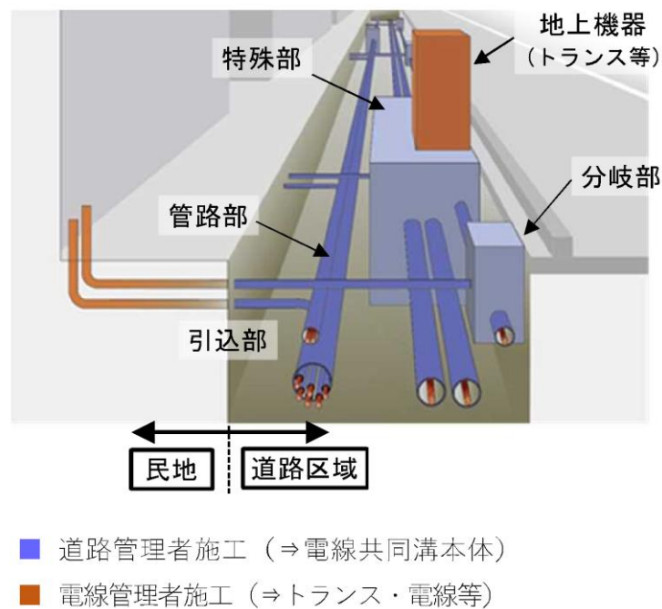
図 1-8 電線共同溝方式のイメージ
