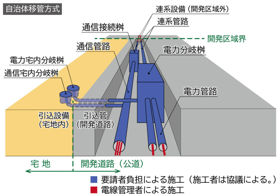
図 1-5 自治体移管方式のイメージ
