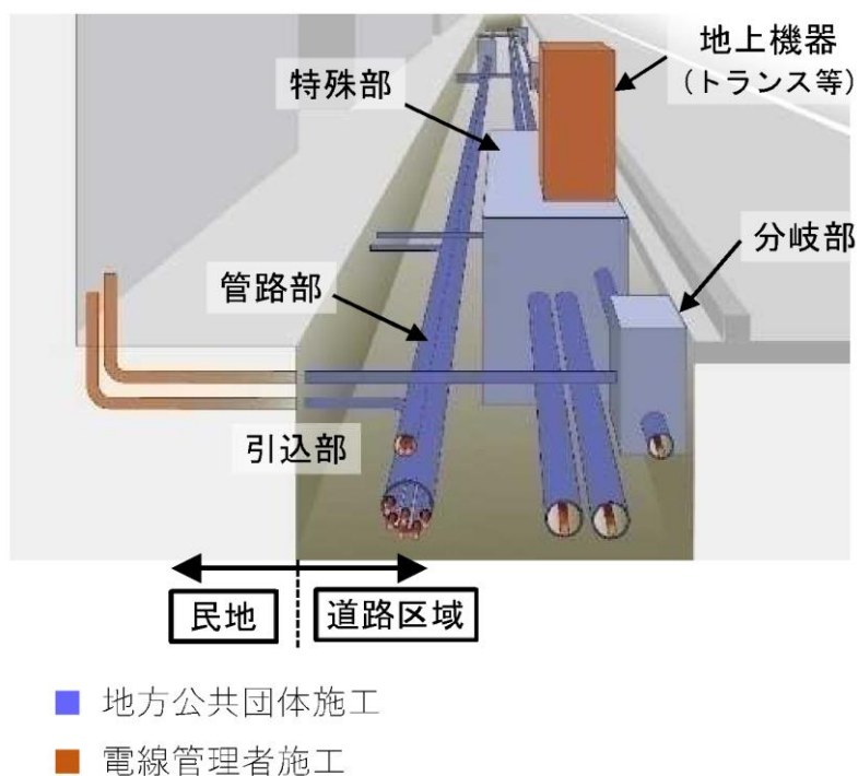
図 1-9 自治体管路方式のイメージ
