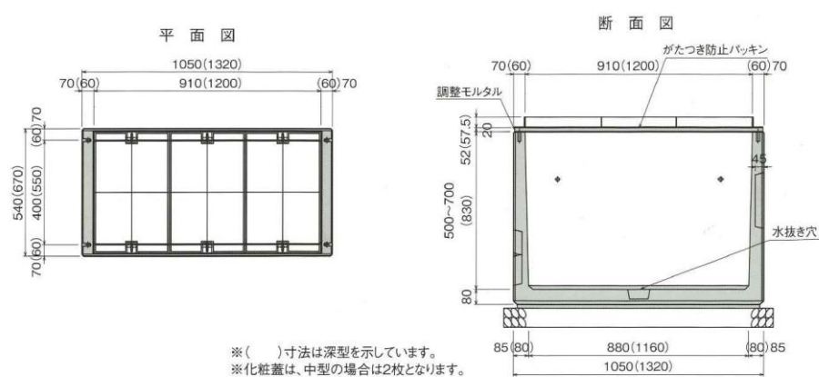
電力宅内分岐櫛の規格
