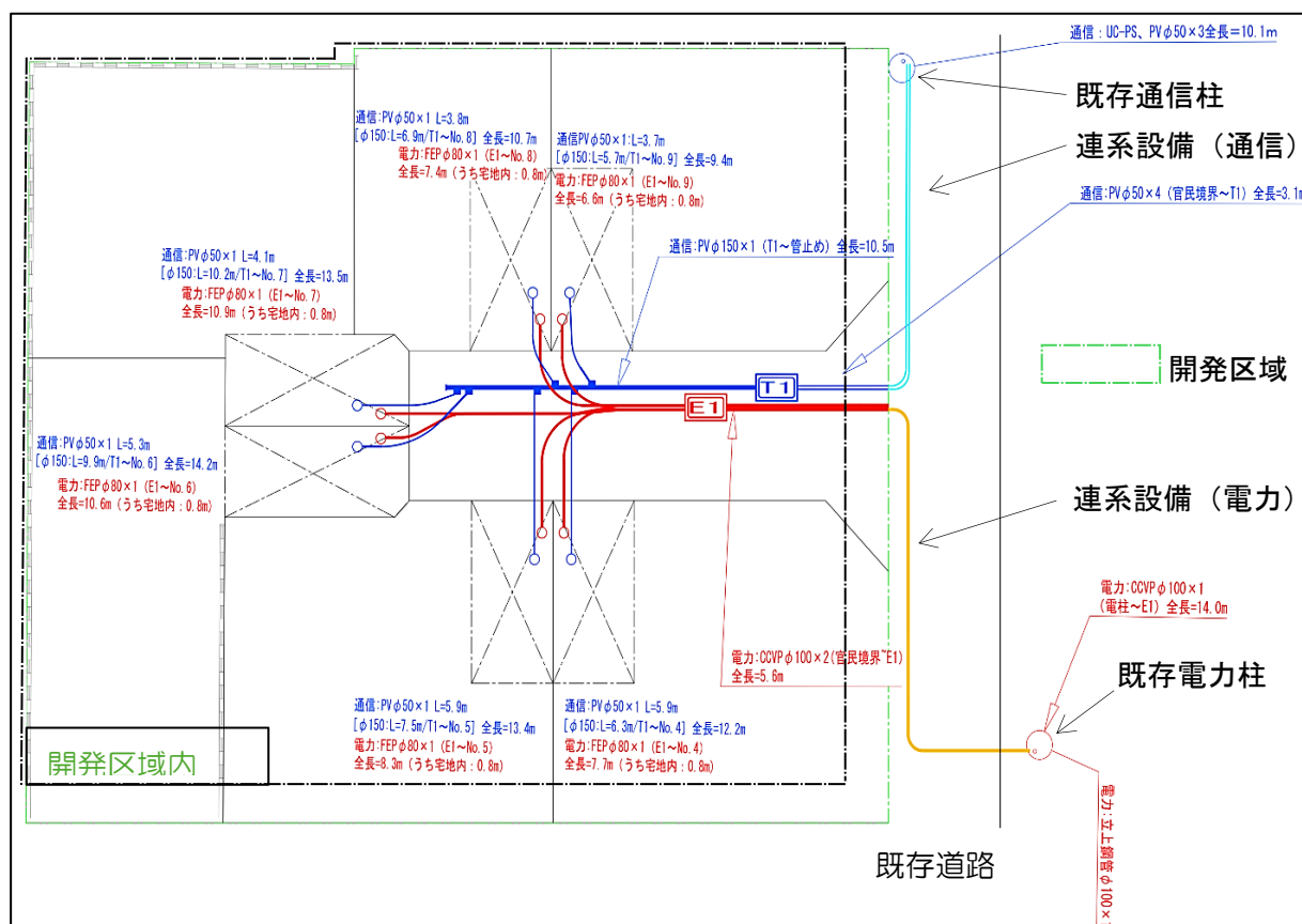
図 2-1 配線計画図の例
