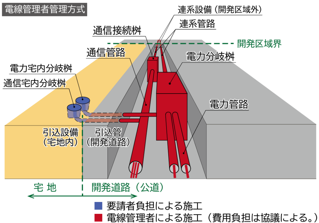
図 1-6 電線管理者方式のイメージ
