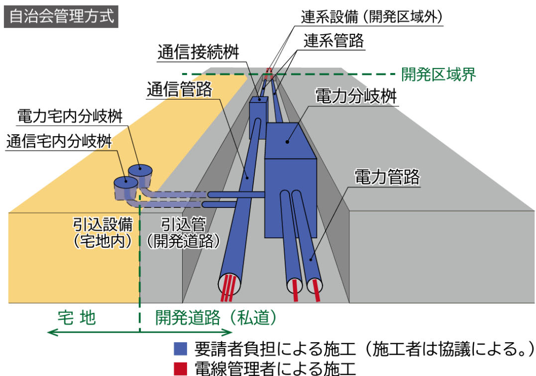
図 1-4 自治会管理方式のイメージ
