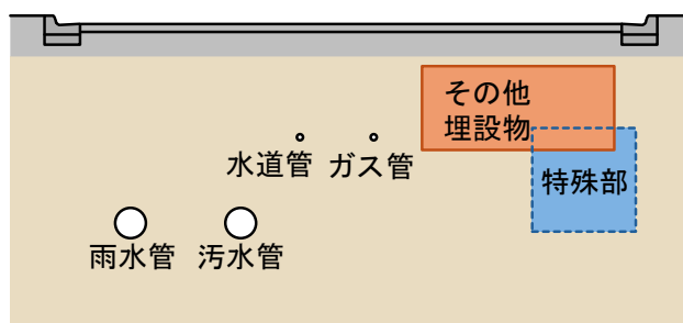
図 - 既に地下に埋設されている占用物件等が多数あり電線を地下に埋設する空間が確保できない場所のイメージ
