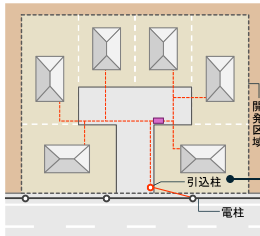
図 - 引込柱として認められる場合
