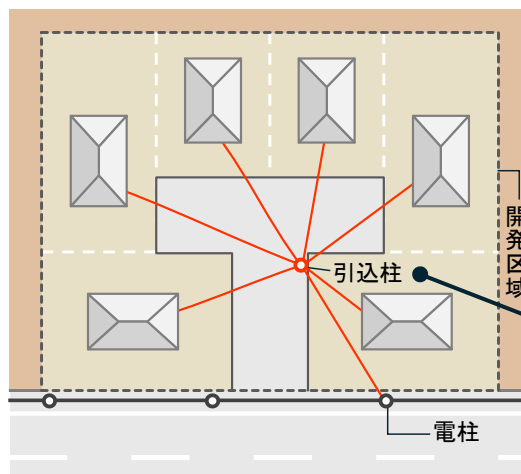
図 - 引込柱として認められない場合
