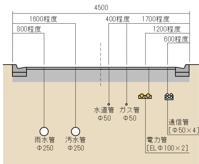
図 - 幅員 4.5m の場合における標準断面図の例
