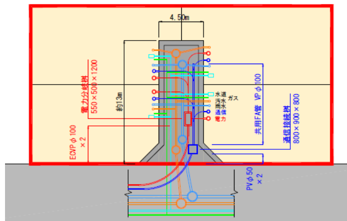
図 - 無電柱化に必要な延長のイメージ
