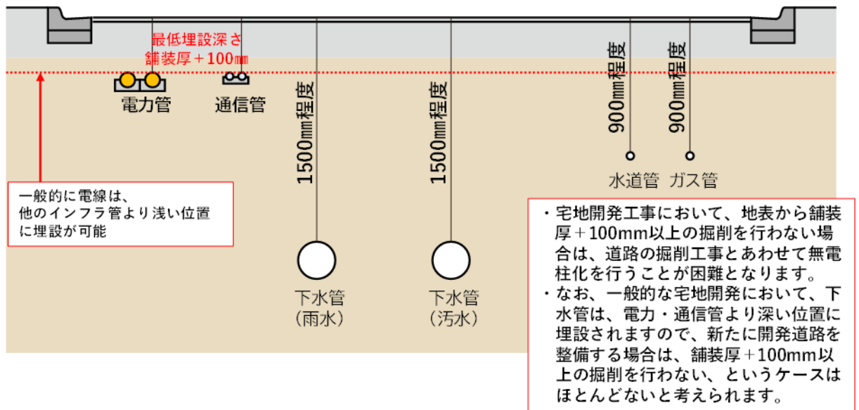
図 - 宅地開発における管路埋設深さの例
