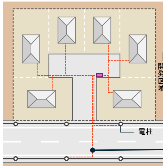
図 - 無電柱化整備
